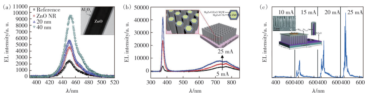
图4 不同注入电流下器件的电致发光谱:(a)ZnO/ \text{Al}_2\text{O}_3 核壳结构 [54] ;(b)MgZnO/ZnO 径向量子阱结构 [34] ;(c)n-ZnO/p-MgZnO 核壳纳米阵列异质结构 [59]
