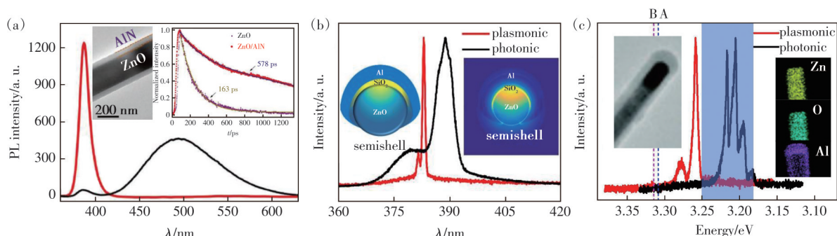
图3 (a)ZnO/AlN核壳结构与纯ZnO纳米线的光致发光与时间分辨荧光光谱 [11] 。等离子体纳米激光器与传统光子激光器的对比:(b)半包裹式Al/SiO 2 /ZnO复合结构 [50] ;(c)全包裹式Al/ZnO复合结构 [28]
