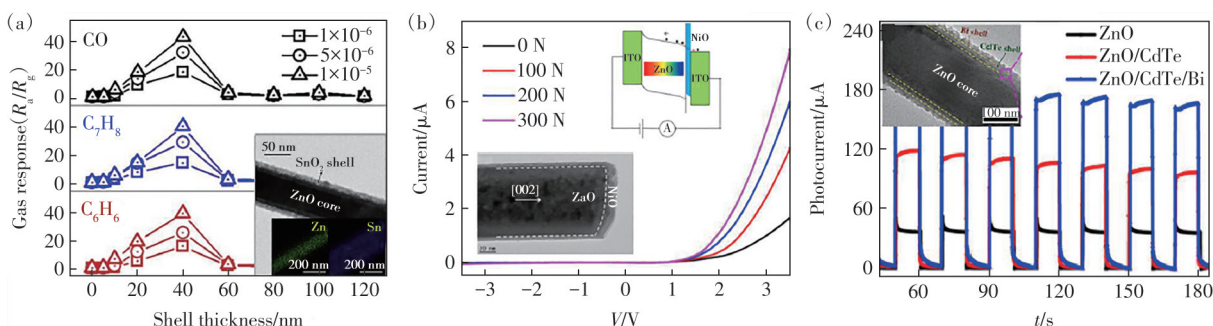
图 8 (a) \text{SnO}_2 壳层厚度与 \text{ZnO}/\text{SnO}_2 核壳结构气体传感响应的关系 [91] ; (b) \text{p-NiO}/\text{n-ZnO} 核壳压力传感器在不同负载条件下的 I - V 特性曲线 [97] ; (c) \text{ZnO}/\text{CdTe}/\text{Bi} 核壳阵列与 \text{ZnO} 、 \text{ZnO}/\text{CdTe} 的光电流对比 [30]
