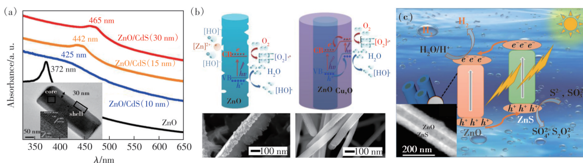
图7 (a)ZnO/CdS核壳结构的吸收光谱 [86] ; (b)ZnO/Cu x O核壳结构与ZnO水稳定性对比 [27] ; (c)ZnO/ZnS核壳异质结构的光催化机制 [90]
