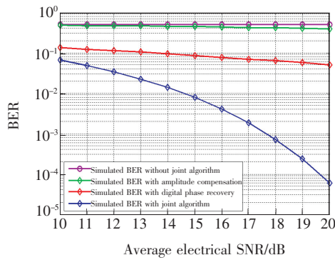
图 7 不同系统的仿真误码率
