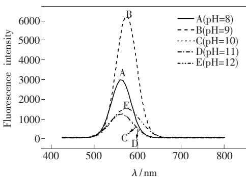
图 3 不同 pH 条件下得到的 CdTe 量子点的荧光发射光谱, 加热温度为 160 °C, 反应时间为 75 min, 激发波长为 360 nm。
