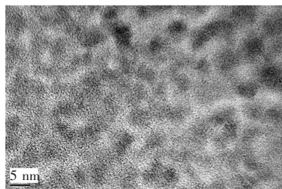
图 5 CdTe 量子点的 TEM 图
