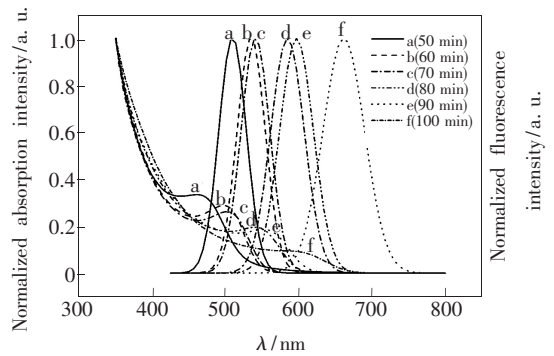
图 1 不同反应时间得到的 CdTe 量子点的紫外-可见吸收光谱和归一化的荧光发射光谱, 加热温度为 160 ^\circ\text{C} , 反应前驱体溶液 pH 值为 10.2, 激发波长为 360 nm。
