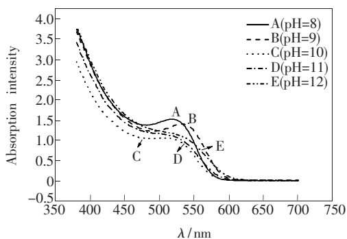
图 2 不同 pH 条件下得到的 CdTe 量子点的紫外-可见吸收光谱, 加热温度为 160 °C, 反应时间为 75 min。
