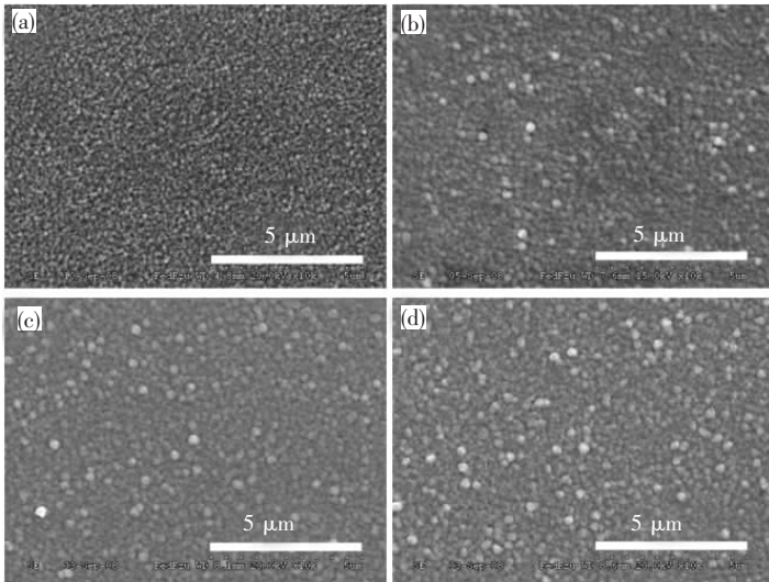
图 3 Ag 膜样品表面的 SEM 图像, 其中 a、b、c 和 d 分别对应于样品 1 # 、4 # 、6 # 和 8 #
